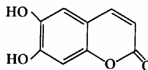
Fig. 7 – Esculetina
