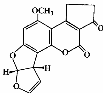
Figura 11 - Aflatoxina B 1
