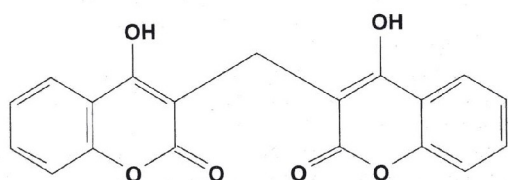
Fig. 9 – Dicumarolo
