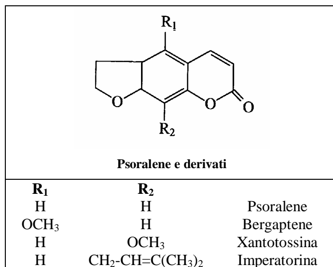
Fig. 10 – Psoraleni
