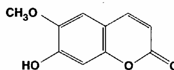
Fig. 8 – Scopoletina
