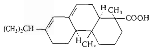
Fig. 6. - Formula di struttura dell'acido abietico.
