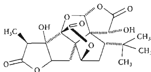
Fig. 4. - Formula di struttura del ginkgolide A.
